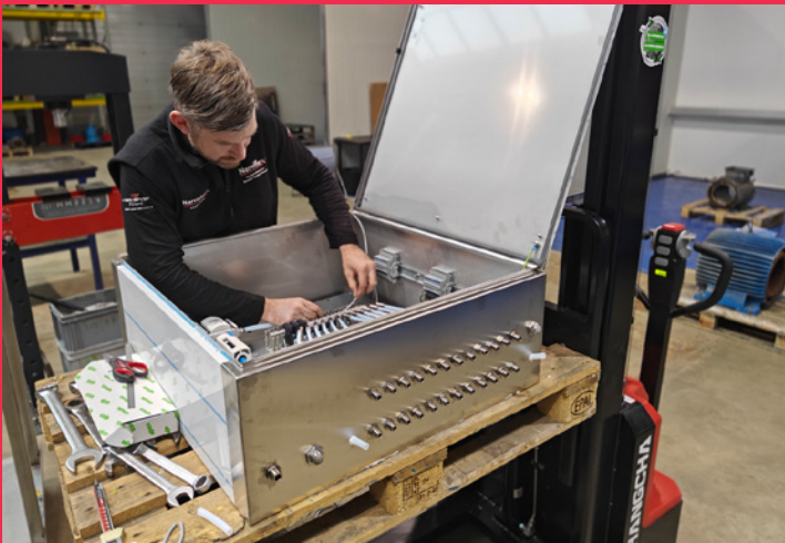
Herstellen, samenstellen en bouwen van perslucht-sturingskasten.
