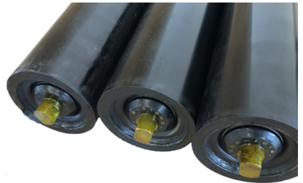
MC-Idler PU, zijkant- en onderrollen standaard met slijtvaste PU bekleed
