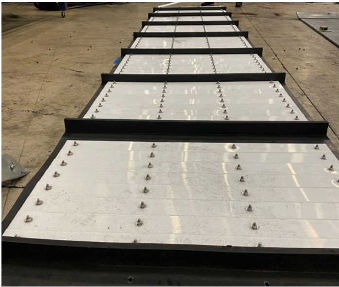
Perfekte samenwerking tussen Narviflex productie van rubber transportbanden en Narviplastx industriële kunststoffen, resulteert in een magneetband met PE 1000 beschermingsstroken.
